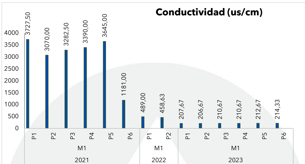
Gráfica 94. Registros de la conductividad en la Ciénaga El Rincón en el monitoreo realizado en julio y agosto de 2023, contrastado con monitoreos anteriores.
