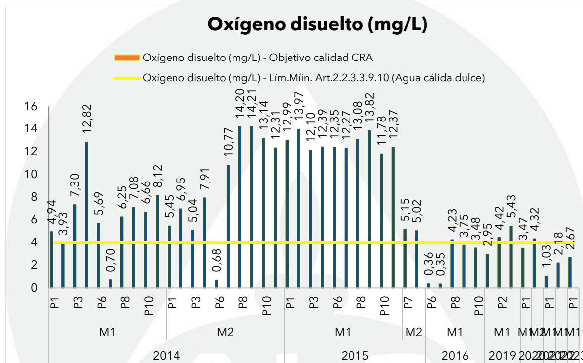
Gráfica 30. Registros de Oxígeno disuelto en la Ciénaga La Luisa julio y agosto de 2023, contrastado con monitoreos anteriores y los objetivos de calidad.
