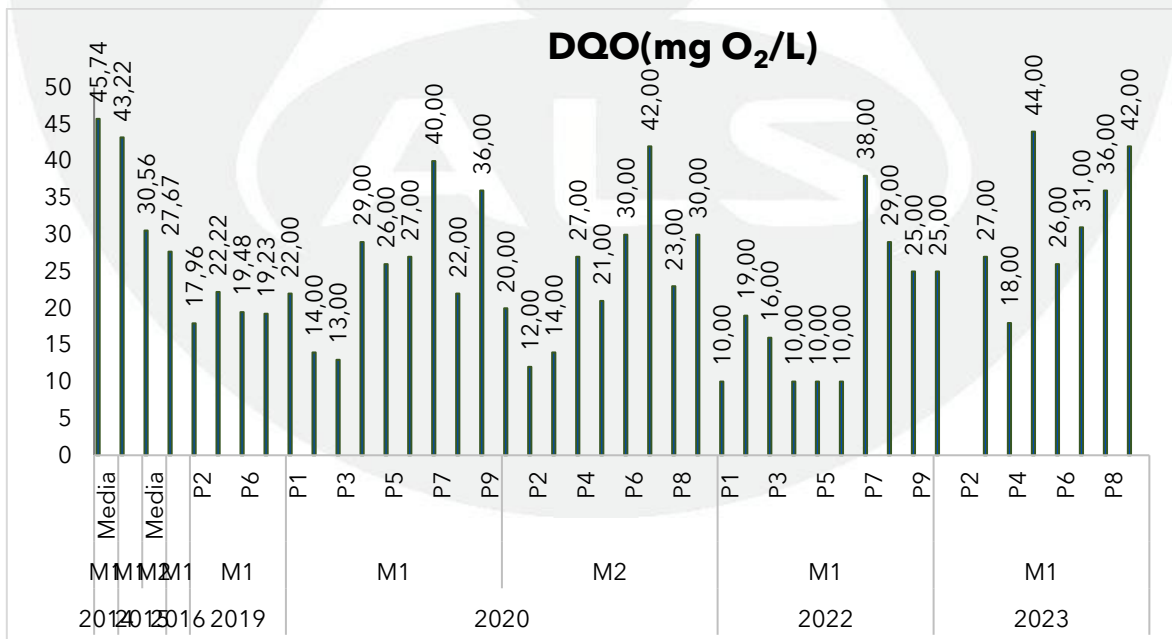
Gráfica 141. Registros de DQO en el Embalse el Guájaró en el monitoreo realizado en julio y agosto de 2023, contrastado con monitoreos anteriores y los objetivos de calidad.
