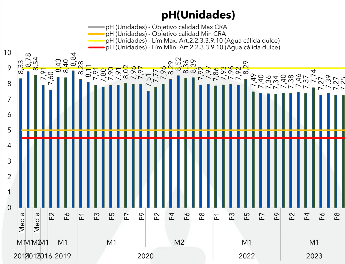
Gráfica 137. Registros del pH en el Embalse el Guájaro en el monitoreo realizado en julio y agosto de 2023 contrastado con monitoreos anteriores y los objetivos de calidad.
