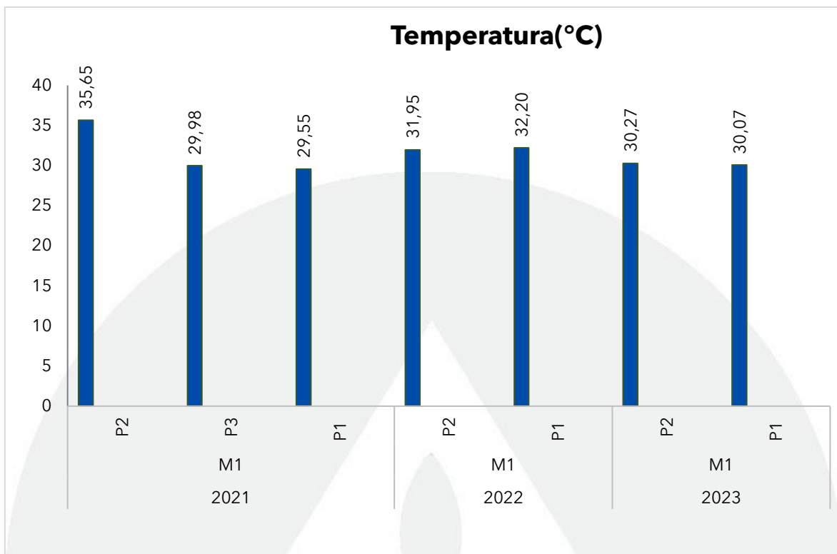
Gráfica 100. Registros de la temperatura en la Ciénaga de Balboa en el monitoreo realizado en julio y agosto de 2023, contrastado con monitoreos anteriores.
