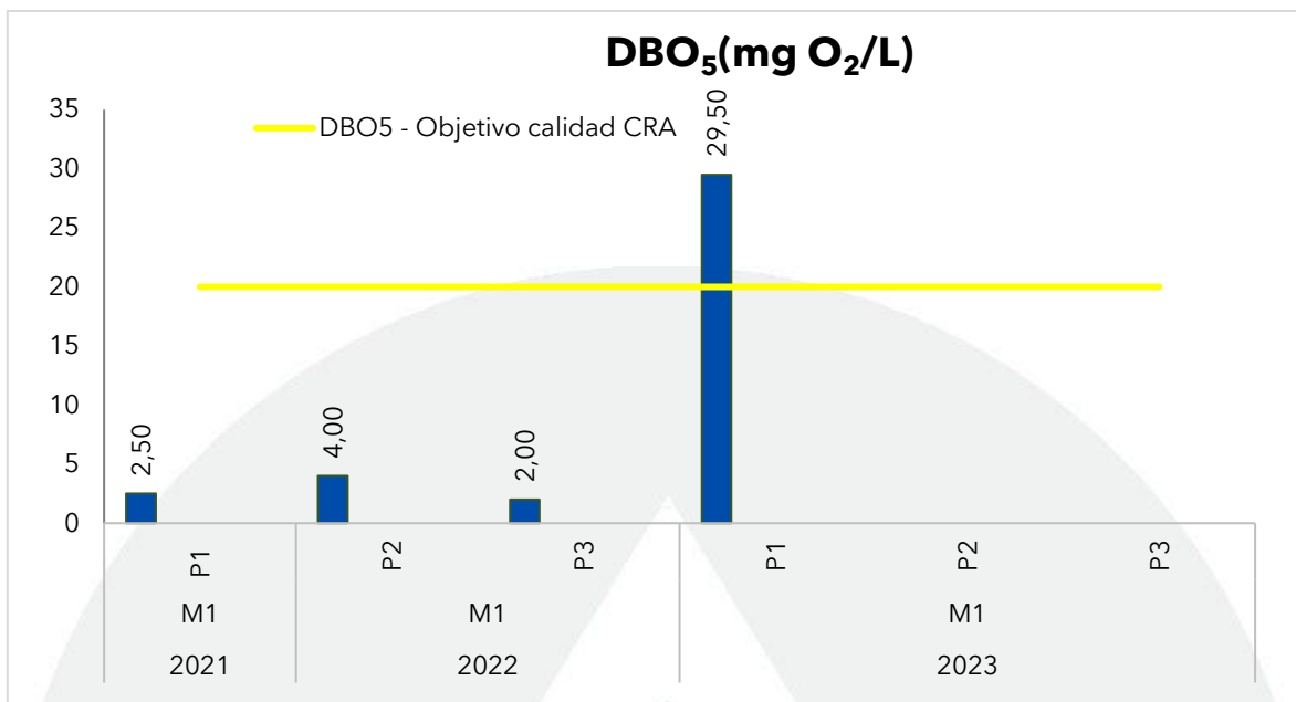
Gráfica 68. Registros de la DBO 5 en el Río Magdalena en el monitoreo realizado en julio y agosto de 2023, contrastado con monitoreos anteriores.
