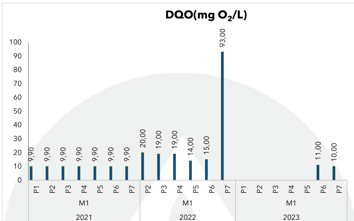
Gráfica 87. Registros de la DQO (mg O 2 /L) en la Ciénaga de Mallorquín en julio y agosto de 2023, contrastado con monitoreos anteriores.
