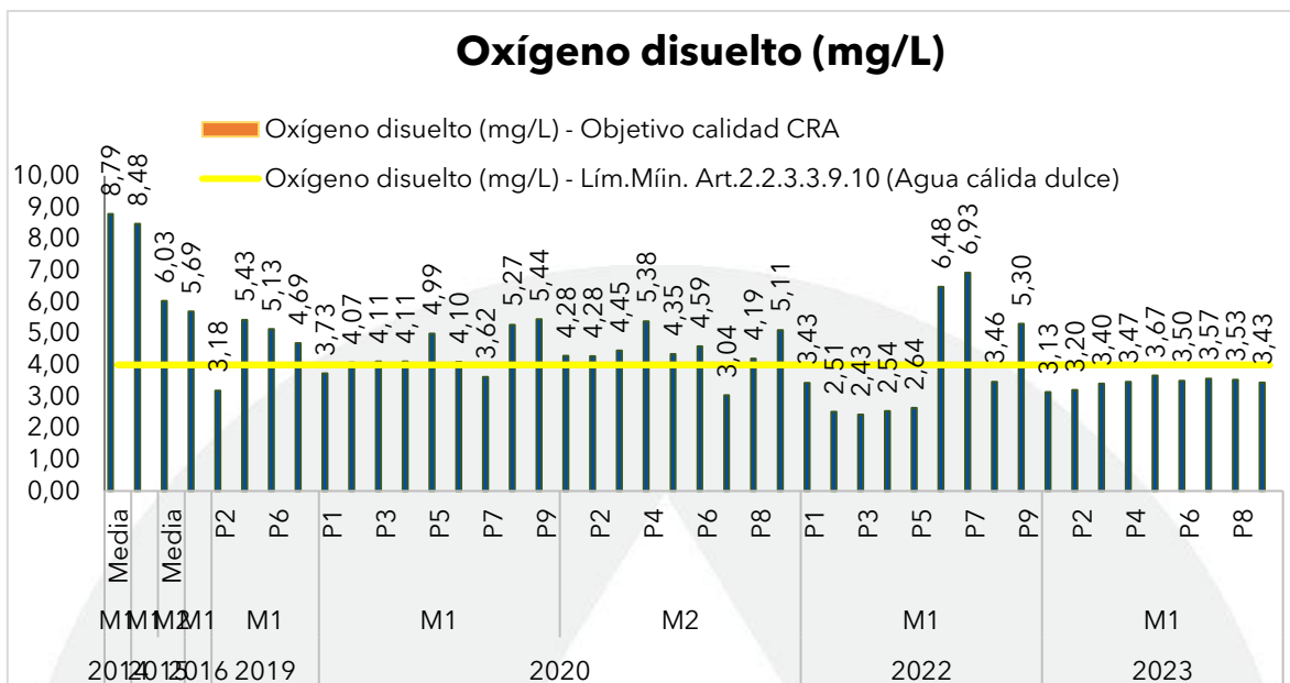
Gráfica 138. Registros del oxígeno disuelto en el Embalse el Guájaro en el monitoreo realizado en julio y agosto de 2023, contrastado con monitoreos anteriores y los objetivos de calidad.
