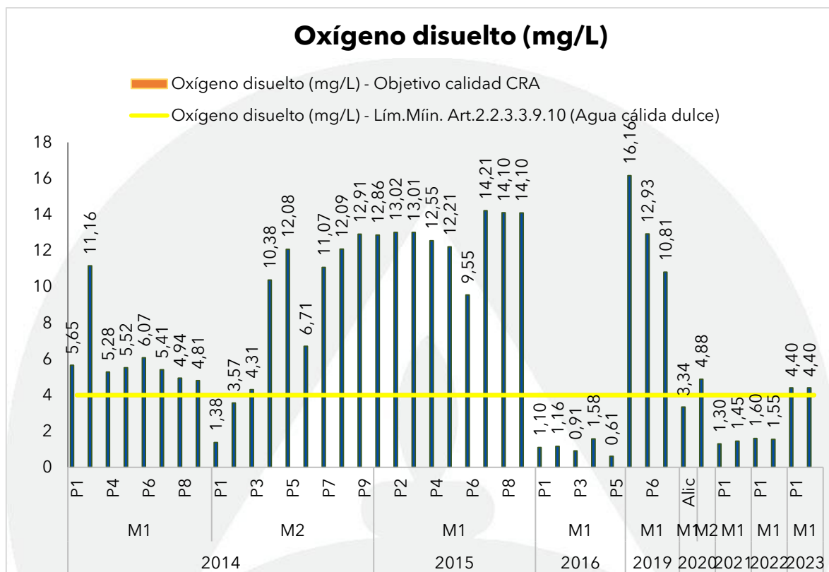
Gráfica 57. Registros del oxígeno disuelto en la Ciénaga de Sabanagrande en julio y agosto de 2023, contrastado con monitoreos anteriores y los objetivos de calidad.
