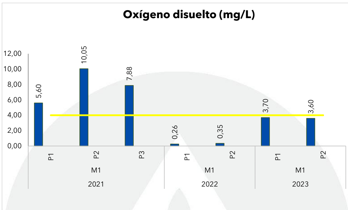
Gráfica 102. Registros del oxígeno disuelto en la Ciénaga de Balboa en el monitoreo en julio y agosto de 2023, contrastado con monitoreos anteriores y los objetivos de calidad.
