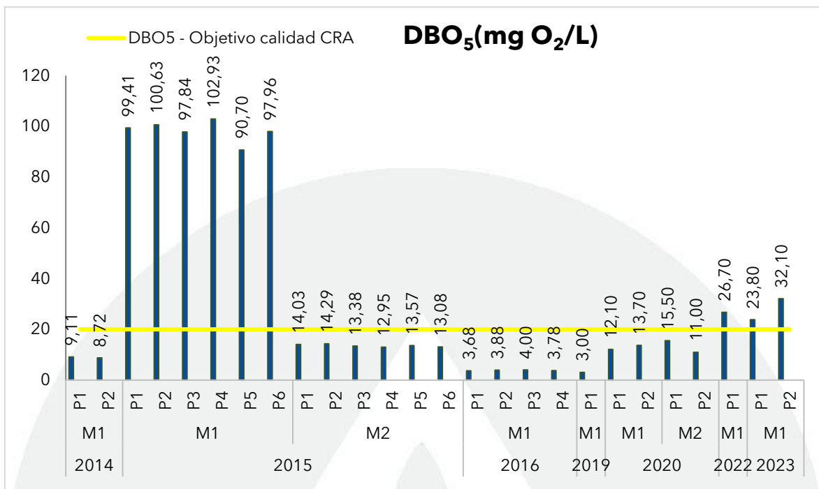
Gráfica 131. Registros de DBO 5 en la Ciénaga San Juan de Tocagua en julio y agosto de 2023, contrastado con monitoreos anteriores y los objetivos de calidad.
