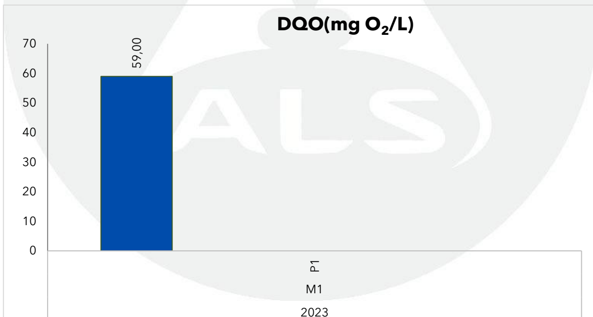
Gráfica 150. Registros de DQO en la Ciénaga Manatí en julio y agosto de 2023, contrastado con monitoreos anteriores.
