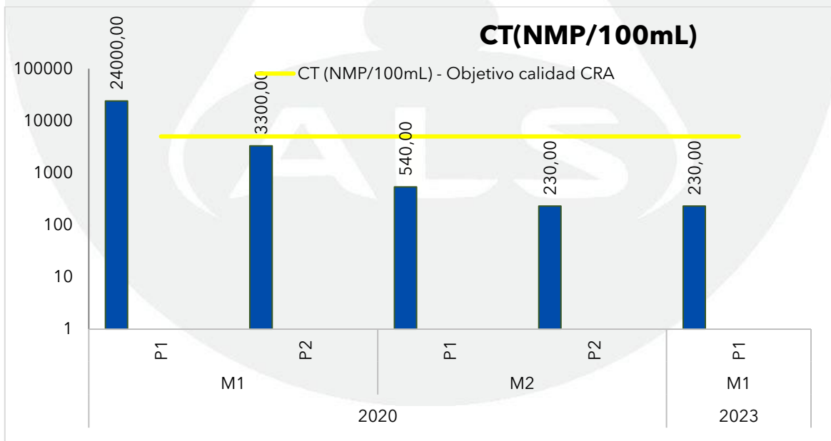
Gráfica 45. Registros de Coliformes Totales (CT) en la Ciénaga La larga en julio y agosto de 2023, contrastado con monitoreos anteriores y los objetivos de calidad.
