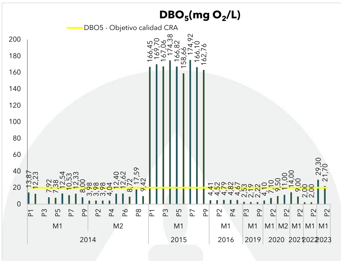
Gráfica 59. Registros de la DBO 5 en la Ciénaga de Sabanagrande en julio y agosto de 2023, contrastado con monitoreos anteriores y los objetivos de calidad.
