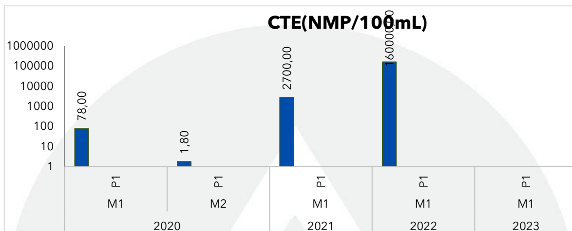
Gráfica 116. Registros de los coliformes termotolerantes (CTE) en la Ciénaga Los Manatíes en el monitoreo realizado en julio y agosto de 2023, contrastado con monitoreos anteriores.
