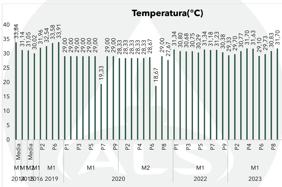
Gráfica 136. Registros de la temperatura en el Embalse el Guájaro en el monitoreo realizado julio y agosto de 2023, contrastado con monitoreos anteriores.
