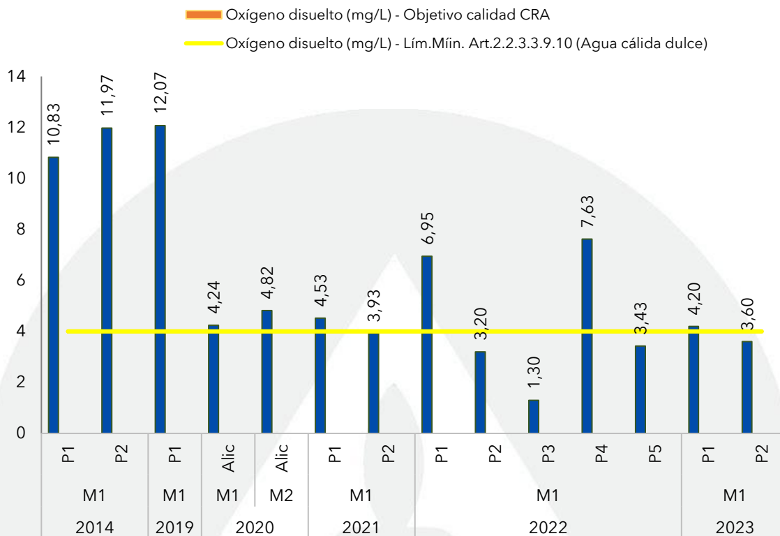
Gráfica 3. Registros del oxígeno disuelto en la Ciénaga de Malambo en julio y agosto de 2023, contrastado con monitoreos anteriores y los objetivos de calidad.
