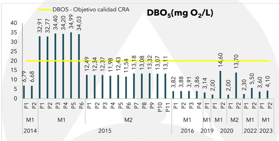
Gráfica 122. Registros de la \text{DBO}_5 en la Ciénaga del Totumo en el monitoreo realizado en julio y agosto de 2023, contrastado con monitoreos anteriores y los objetivos de calidad.
