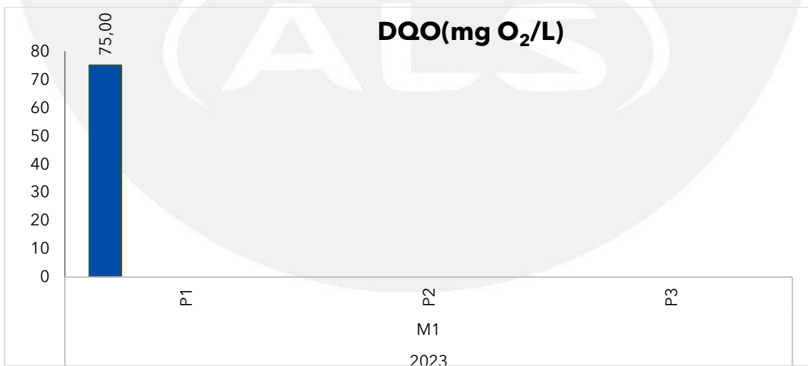
Gráfica 69. Registros de la DQO en el Río Magdalena en el monitoreo realizado en julio y agosto de 2023, contrastado con monitoreos anteriores.
