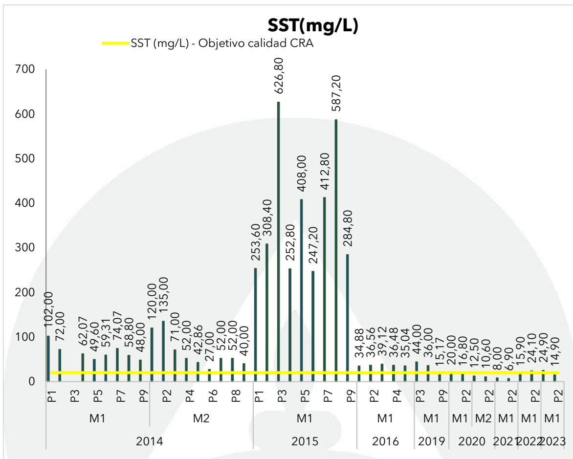
Gráfica 61. Registros de SST en la Ciénaga de Sabanagrande en julio y agosto de 2023, contrastado con monitoreos anteriores y los objetivos de calidad.
