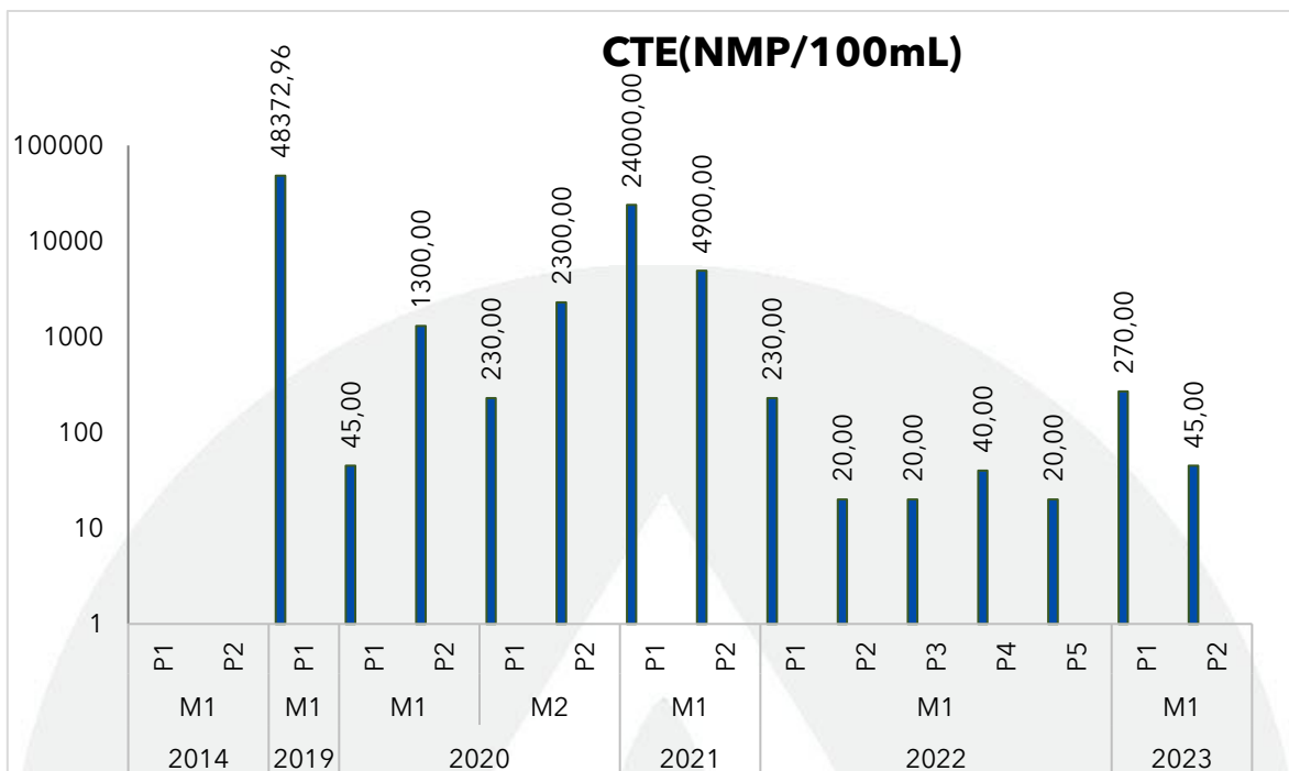
Gráfica 8. Registros de coliformes termotolerantes (CTE) en la Ciénaga de Malambo en julio y agosto de 2023, contrastado con monitoreos anteriores
