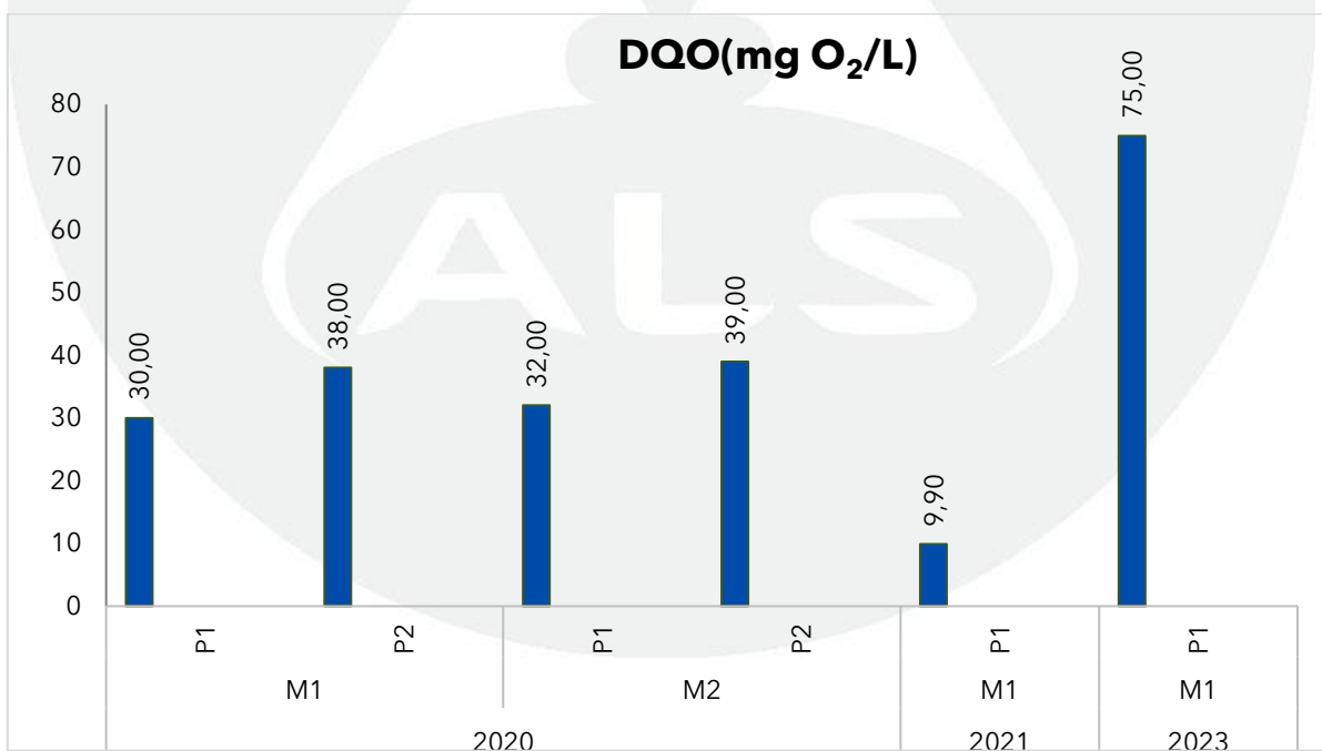
Gráfica 78. Registros de la DQO en la Ciénaga Paraíso en el monitoreo realizado en julio y agosto de 2023, contrastado con monitoreos anteriores.
