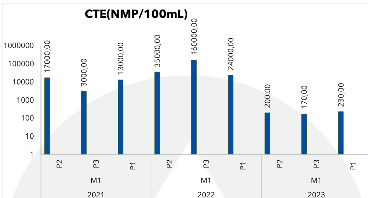
Gráfica 71. Registros de coliformes termotolerantes (CTE) en el Río Magdalena en el monitoreo realizado en julio y agosto de 2023, contrastado con monitoreos anteriores.
