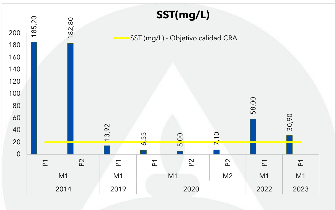
Gráfica 52. Registros de SST en la Ciénaga El Uvero en julio y agosto de 2023, contrastado con monitoreos anteriores y los objetivos de calidad.
