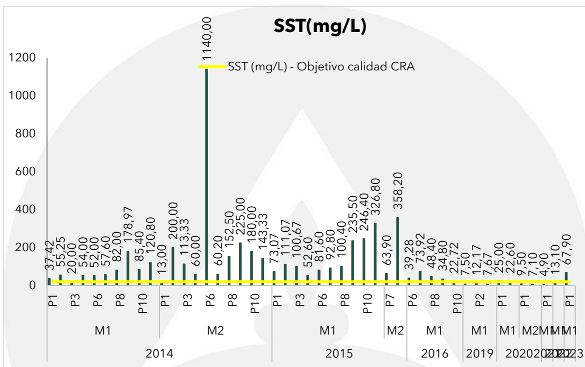
Gráfica 34. Registros de SST en la en la Ciénaga La Luisa en julio y agosto de 2023, contrastado con monitoreos anteriores y los objetivos de calidad.
