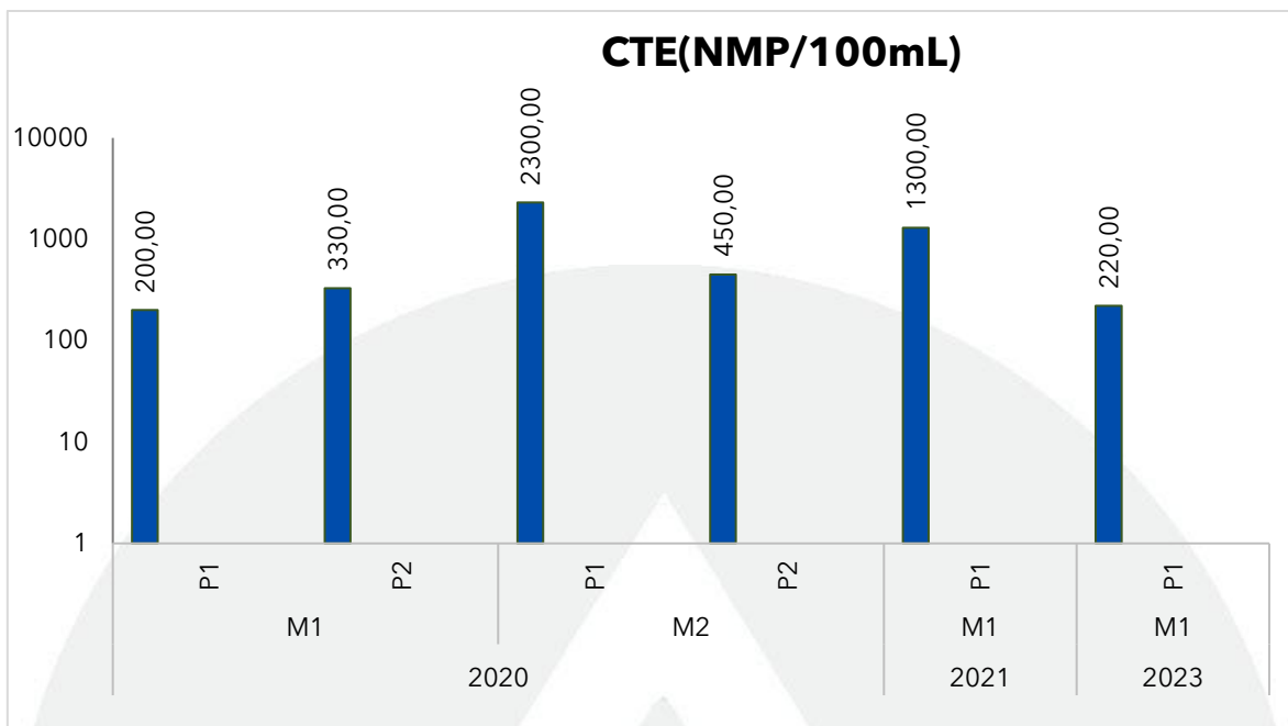
Gráfica 80. Registros de los coliformes termotolerantes (CTE) en la Ciénaga Paraíso en el monitoreo realizado en julio y agosto de 2023, contrastado con monitoreos anteriores.
