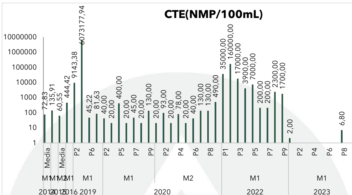
Gráfica 143. Registros de coliformes termotolerantes (CTE) en el Embalse el Guájaro en el monitoreo realizado julio y agosto de 2023, contrastado con monitoreos anteriores.
