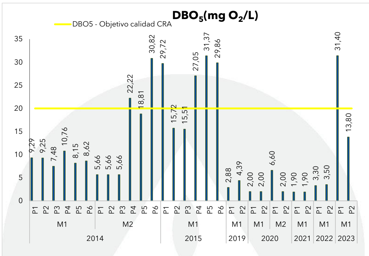
Gráfica 23. Registros de la DBO 5 en la Ciénaga de Santo Tomás en el monitoreo realizado en julio y agosto de 2023, contrastado con monitoreos anteriores y los objetivos de calidad.
