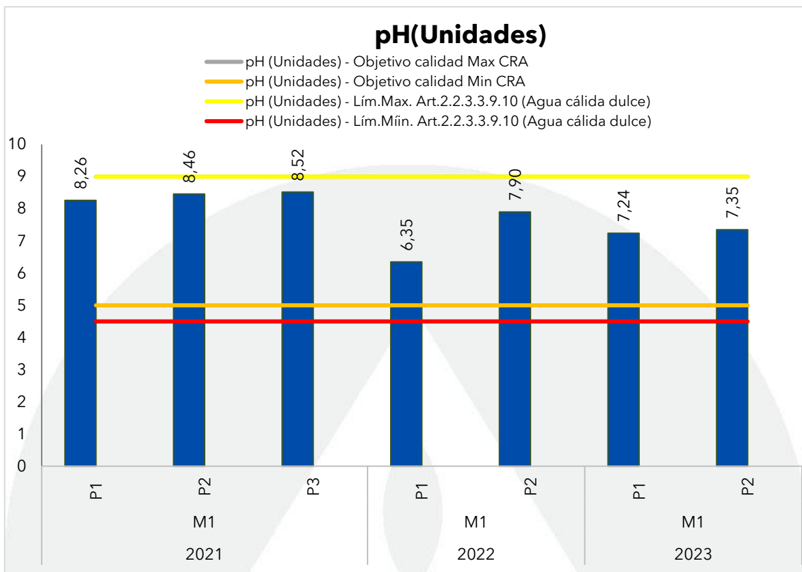
Gráfica 101. Registros del pH en la Ciénaga de Balboa en el monitoreo realizado en julio y agosto de 2023, contrastado con monitoreos anteriores y los objetivos de calidad.
