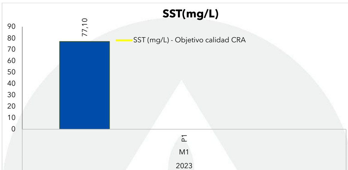
Gráfica 151. Registros de SST en la Ciénaga Manatí en julio y agosto de 2023, contrastado con monitoreos anteriores y los objetivos de calidad.
