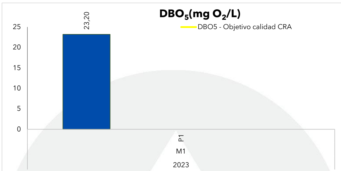
Gráfica 149. Registros de DBO 5 en la Ciénaga Manatí en julio y agosto de 2023, contrastado con monitoreos anteriores y los objetivos de calidad.
