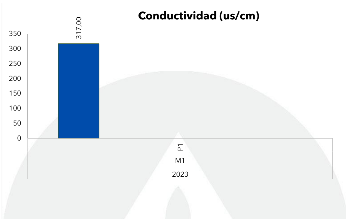
Gráfica 31. Registros de Conductividad en la Ciénaga La Luisa en julio y agosto de 2023, contrastado con monitoreos anteriores.
