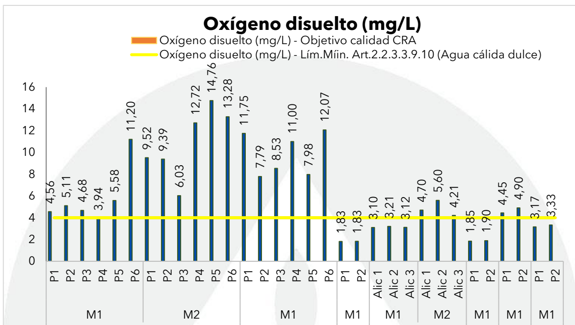
Gráfica 21. Registros del oxígeno disuelto en la Ciénaga de Santo Tomás en el monitoreo realizado en julio y agosto de 2023, contrastado con monitoreos anteriores y los objetivos de calidad.
