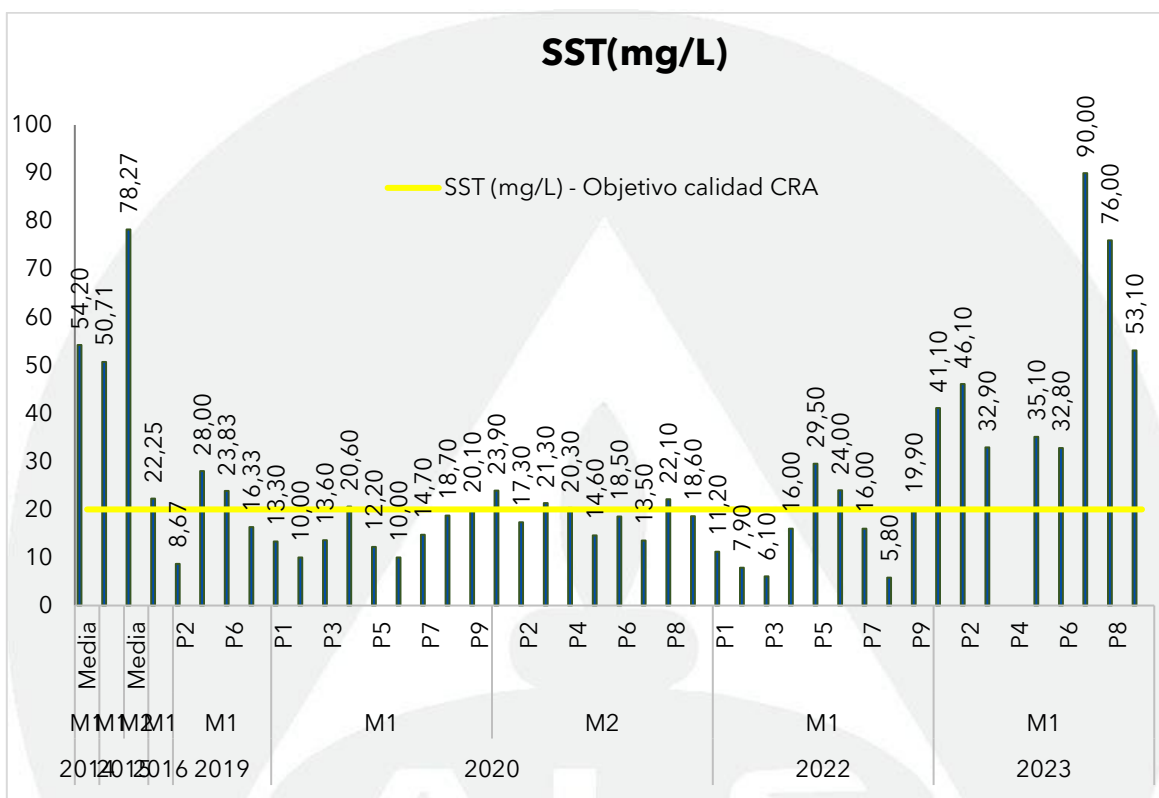
Gráfica 142. Registros de SST en el Embalse el Guájaro en el monitoreo realizado en julio y agosto de 2023 contrastado con monitoreos anteriores y los objetivos de calidad.
