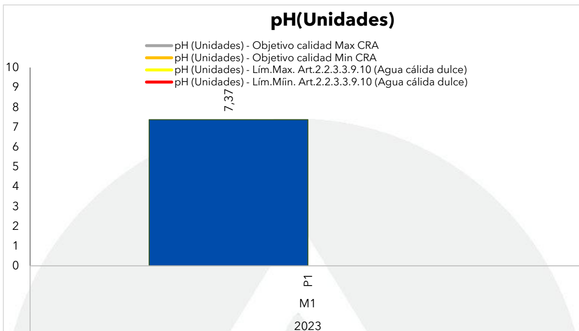
Gráfica 146. Registros de pH en la Ciénaga Manatí en julio y agosto de 2023, contrastado con monitoreos anteriores y los objetivos de calidad.
