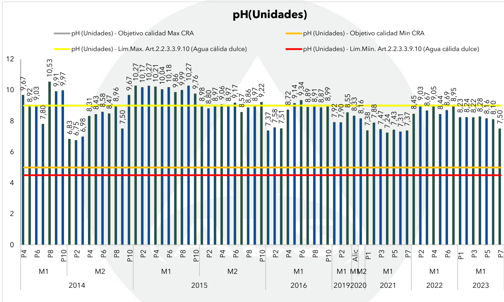
Gráfica 83. Registros del pH (Unidades) en la Ciénaga de Mallorquín en julio y agosto de 2023, contrastado con monitoreos anteriores y los objetivos de calidad.
