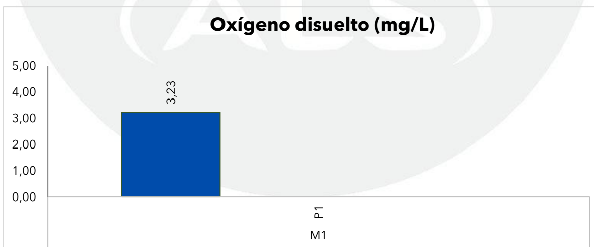
Gráfica 147. Registros de oxígeno disuelto en la Ciénaga Manatí en julio y agosto de 2023, contrastado con monitoreos anteriores y los objetivos de calidad.
