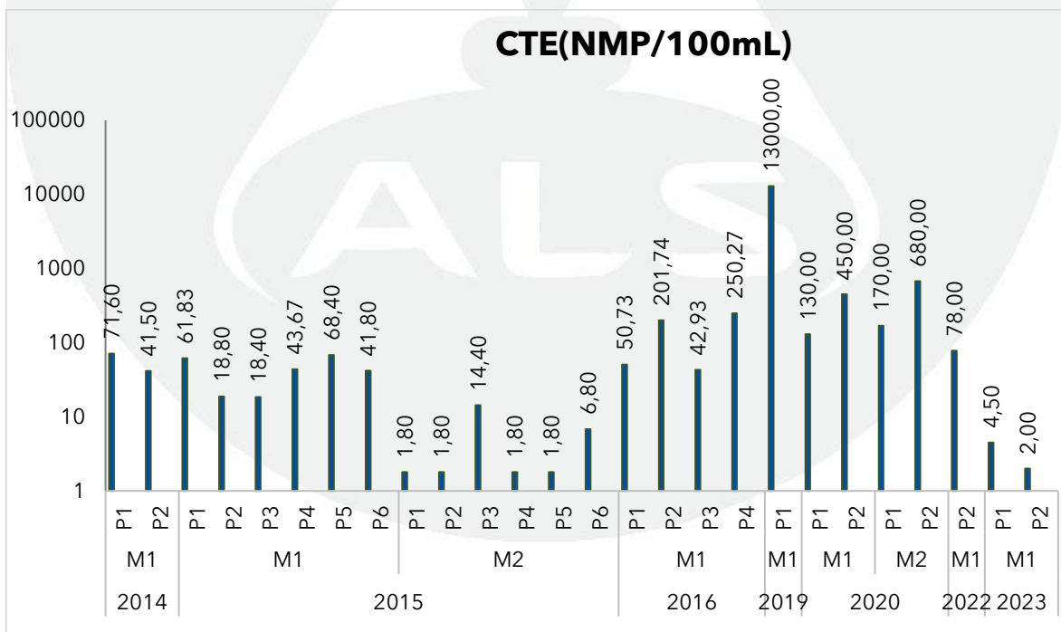
Gráfica 135. Registros de Coliformes termotolerantes (CTE) en la Ciénaga San Juan de Tocagua en julio y agosto de 2023, contrastado con los monitoreos anteriores.
