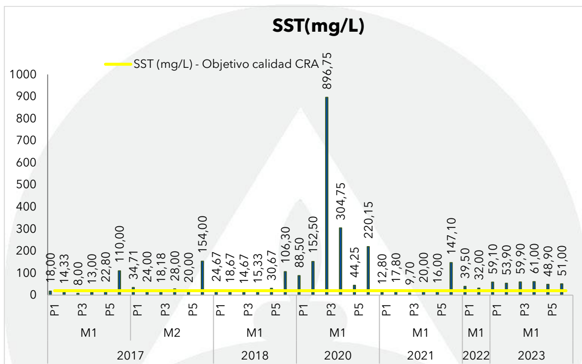
Gráfica 97. Registros de SST en la Ciénaga El Rincón en el monitoreo realizado en julio y agosto de 2023, contrastado con monitoreos anteriores y los objetivos de calidad.
