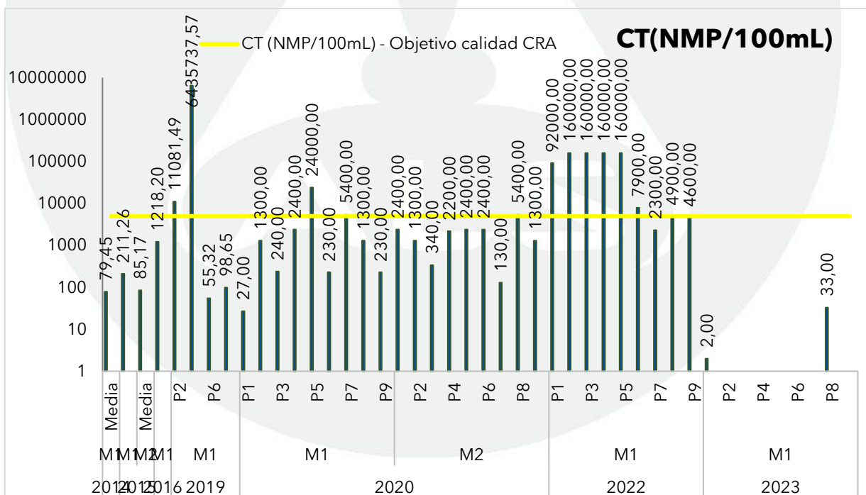
Gráfica 144. Registros de coliformes Totales (CT) en el Embalse el Guájaro en el monitoreo realizado en julio y agosto de 2023, contrastado con monitoreos anteriores y los objetivos de calidad.
