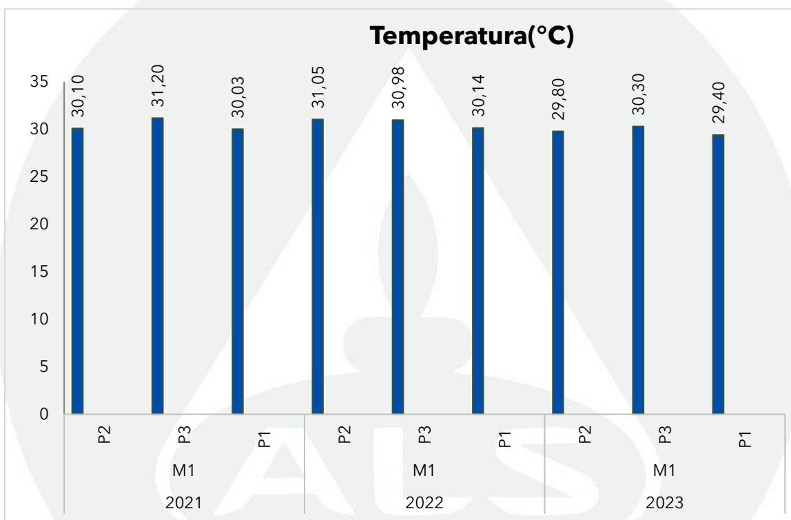
Gráfica 64. Registros de la temperatura en el Río Magdalena en el monitoreo realizado en octubre de 2022, contrastado con monitoreos anteriores y los objetivos de calidad.
