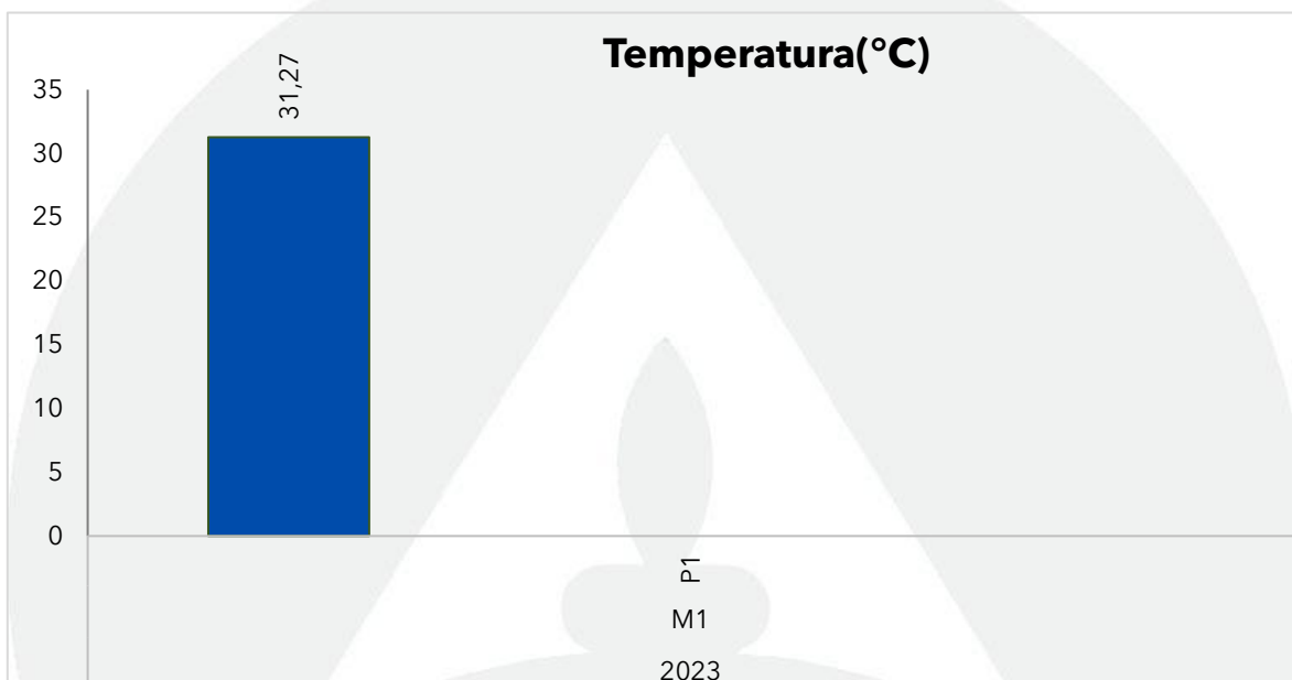
Gráfica 145. Registros de temperatura (°C) en la Ciénaga de Manatí en julio y agosto de 2023, contrastado con monitoreos anteriores.
