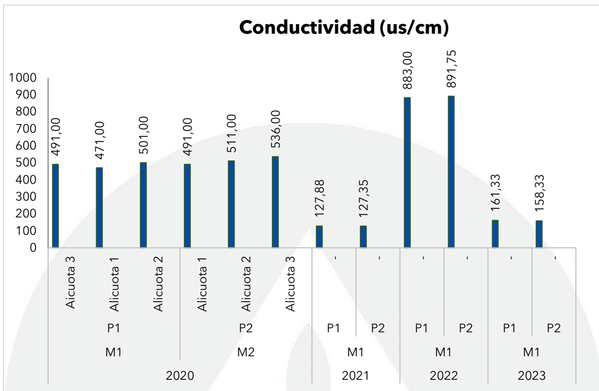
Gráfica 13. Registros de la conductividad en la Ciénaga de Mesolandia en julio y agosto de 2023, contrastado con monitoreos anteriores y los objetivos de calidad.
