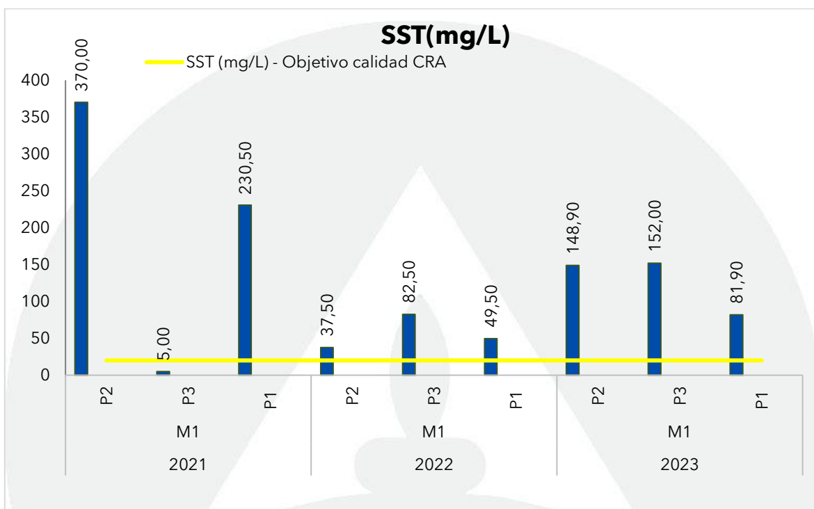
Gráfica 70. Registros de SST en el Río Magdalena en el monitoreo en julio y agosto de 2023, contrastado con monitoreos anteriores y los objetivos de calidad.
