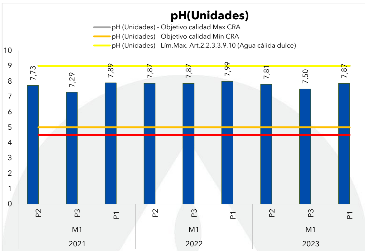
Gráfica 65. Registros del pH en el Río Magdalena en el monitoreo realizado en julio y agosto de 2023, contrastado con monitoreos anteriores y los objetivos de calidad.
