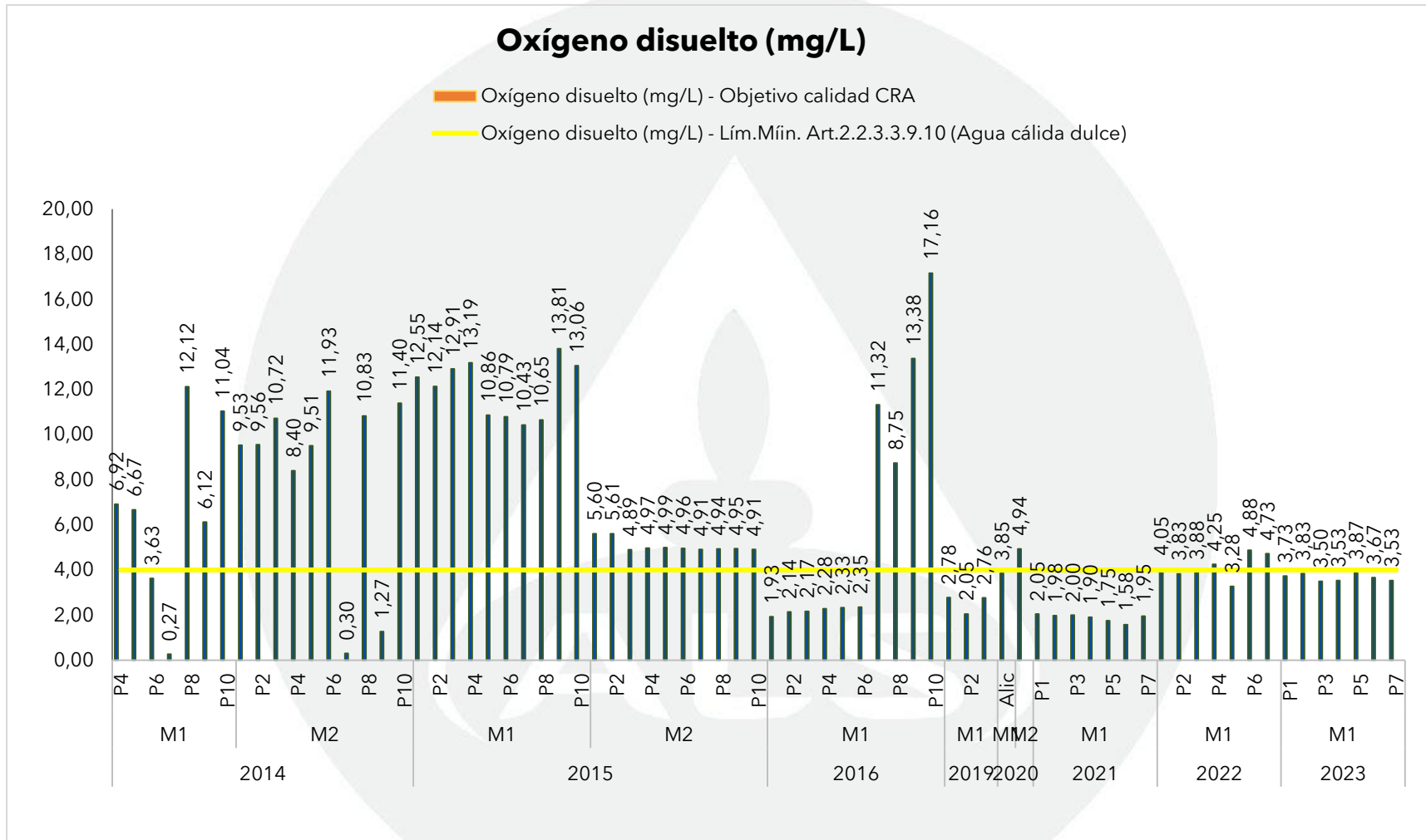
Gráfica 84. Registros del oxígeno disuelto (mg/L) en la Ciénaga de Mallorquín en julio y agosto de 2023, contrastado con monitoreos anteriores y los objetivos de calidad.
