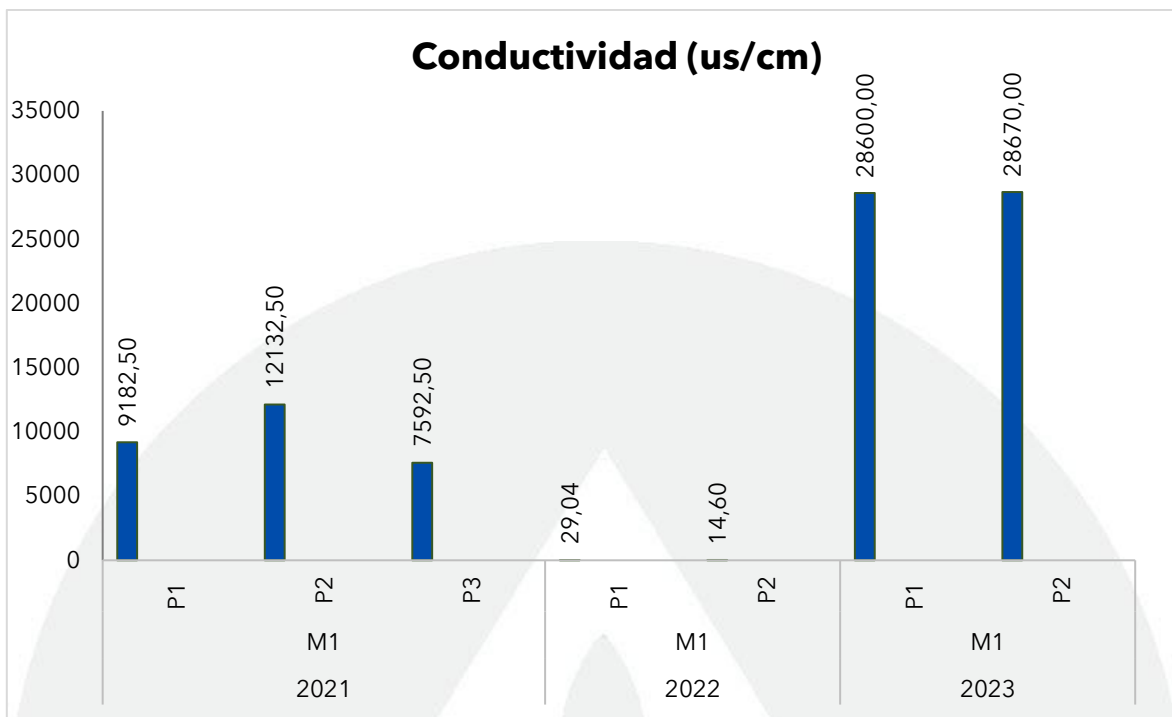
Gráfica 103. Registros de la conductividad en la Ciénaga de Balboa en el monitoreo realizado en julio y agosto de 2023, contrastado con monitoreos anteriores.
