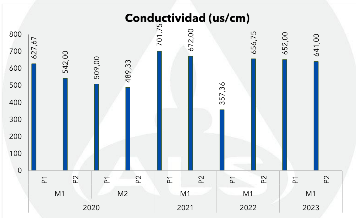
Gráfica 121. Registros de la conductividad en la Ciénaga del Totumo en el monitoreo realizado en julio y agosto de 2023, contrastado con monitoreos anteriores y los objetivos de calidad.
